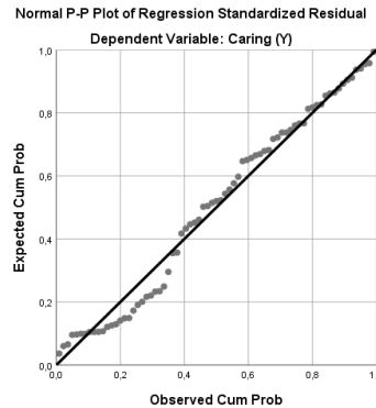
Gambar 1 Grafik Ploting Pada Uji Normalitas
